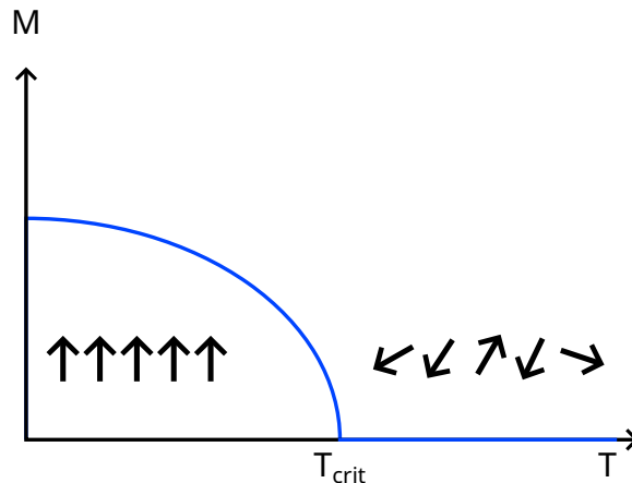
Εικόνα 1: Γραφική αναπαράσταση της παραμέτρου τάξης ( M ) σε σχέση με τη θερμοκρασία σε μια μετάβαση φάσης. Κάτω από την κρίσιμη θερμοκρασία T_{crit} η παράμετρος τάξης αυξάνεται και είναι μη μηδενική, ενώ είναι ίση με μηδέν σε θερμοκρασίες μεγαλύτερες της T_{crit} .
