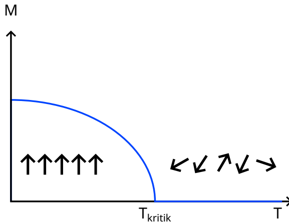
Şekil-1: Düzen parametresinin M faz geçişinde sıcaklığa bağlılığının şematik gösterimi. T_{\text{crit}} kritik sıcaklığının altındayken düzen parametresi artmaktadır (sıfır değildir). T_{\text{crit}} değerinden büyükken ise bu değer sıfıra eşittir.
