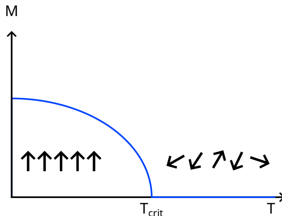
圖 1：相變過程中「序參數」 M 隨溫度變化的示意圖。當低於臨界溫度 T_{\text{crit}} 時，系統的序參數會隨溫度的降低而變大，反之當高於臨界溫度 T_{\text{crit}} 時，系統的序參數等於零。
